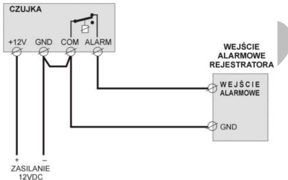
Rys. 3-7. Schemat podłączenia czujek do wejść alarmowych rejestratora.
