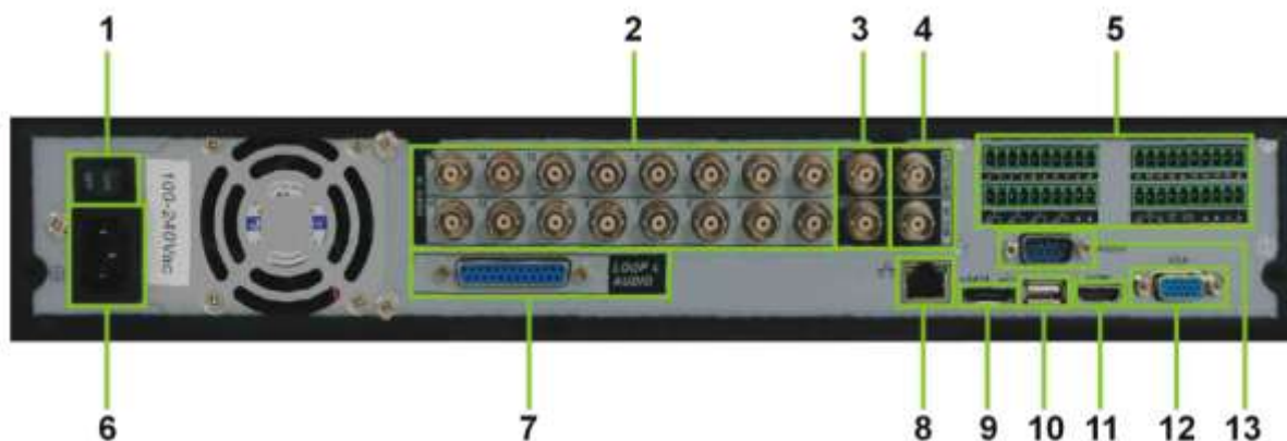
Rysunek 2-2a. Wygląd tylnego panela rejestratora 16-kanalowego serii LE-L.
