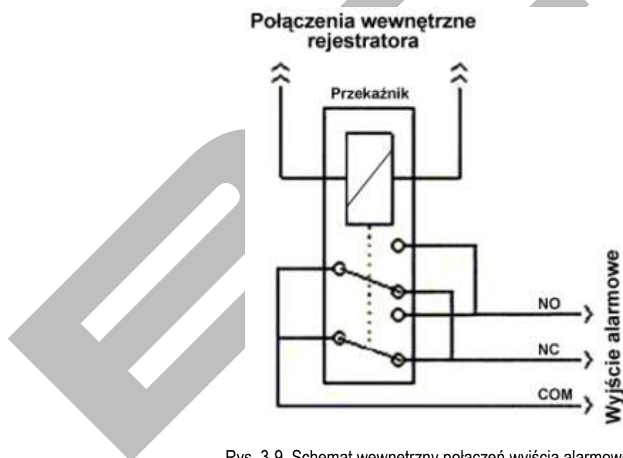
Rys. 3-9. Schemat wewnętrzny połączeń wyjścia alarmowego.
