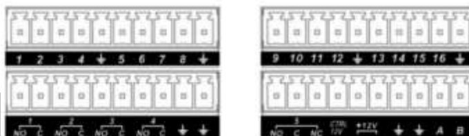
Rys. 3-6a. Rozmieszczenia wejść / wyjść alarmowych rejestratora 16 kanałowego serii LE-L.
