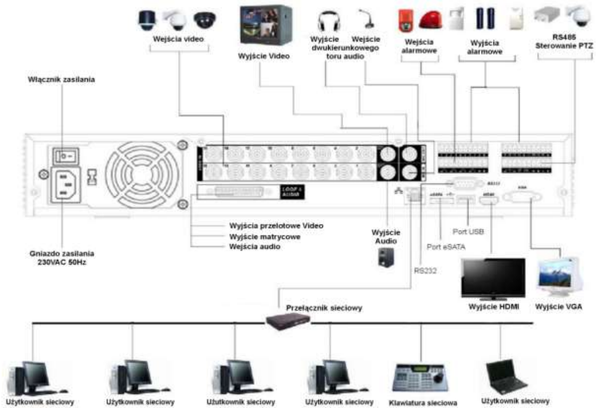
Rysunek 2-3a. Przykładowy schemat podłączenia urządzeń peryferyjnych do rejestratora serii LE-L.
