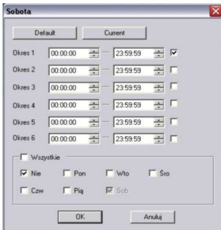
Rys. 7-38b. Ustawianie terminarza aktywności wejścia alarmowego.
