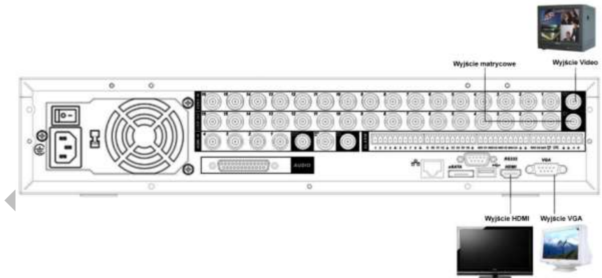
Rys. 3-2. Podłączenie monitorów do rejestratora.
