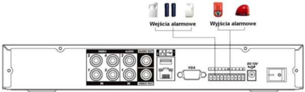
Rys. 3-4b. Podłączenie wejść i wyjść alarmowych w rejestratorach. serii LE-AS.
