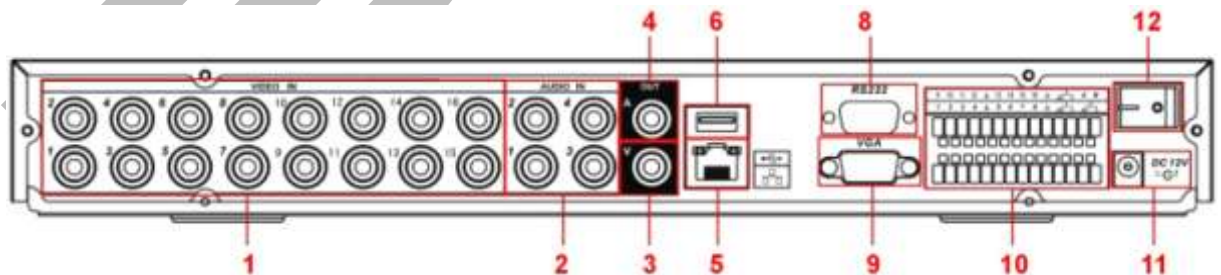
Rysunek 2-3c. Wygląd tylnego panelu rejestratora 16-kanałowego serii LE-AS.
