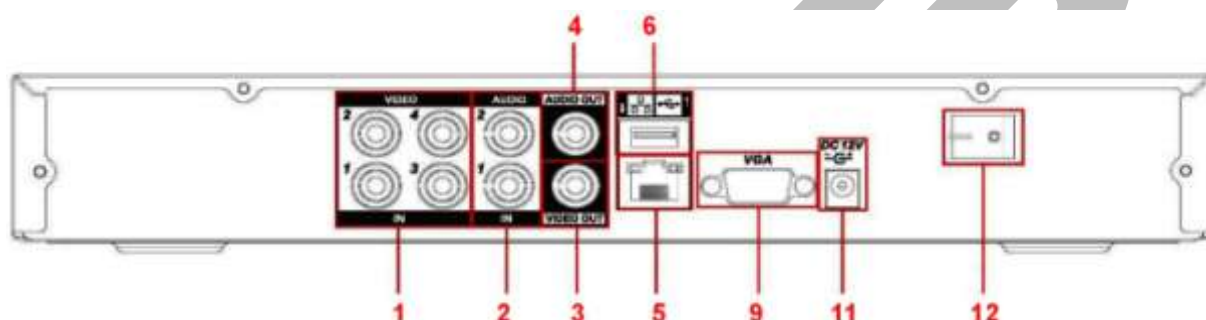
Rysunek 2-4. Wygląd tylnego panelu rejestratora 4-kanałowego serii LE-AN.
