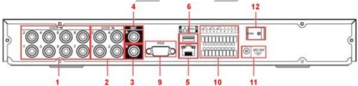
Rysunek 2-3b. Wygląd tylnego panelu rejestratora 8-kanałowego serii LE-AS.
