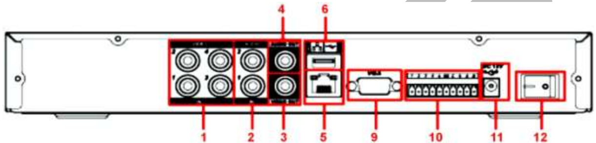
Rysunek 2-3a. Wygląd tylnego panelu rejestratora 4-kanałowego serii LE-AS.
